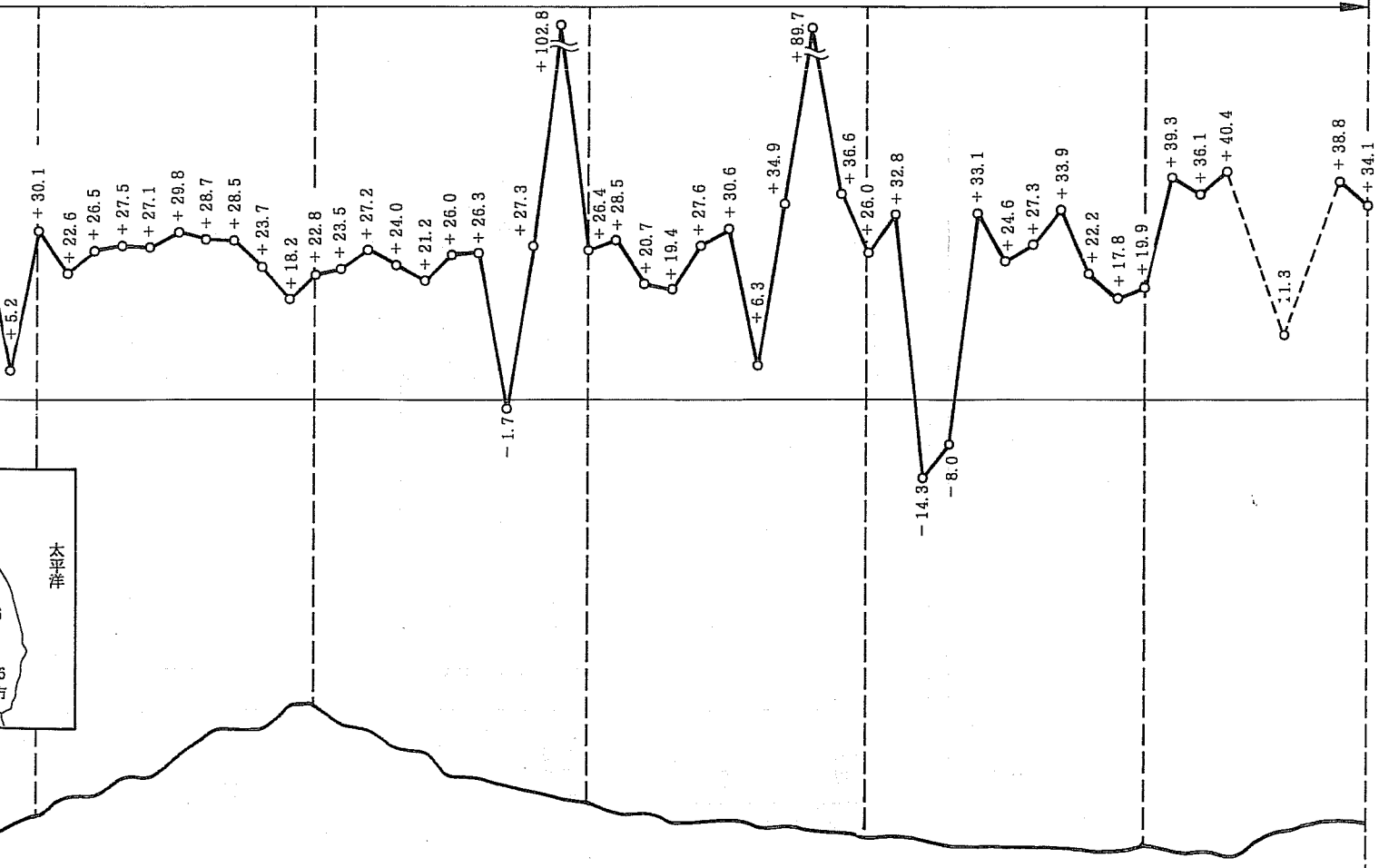
点标高断面图
