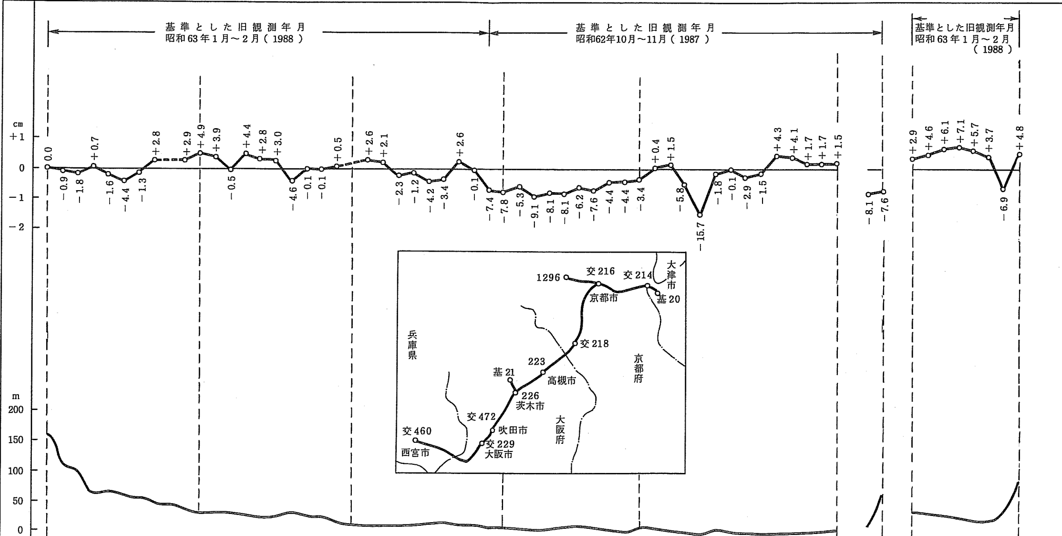
水准点標高断面図
