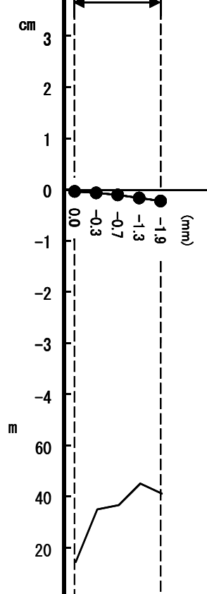
水準点標高断面図
