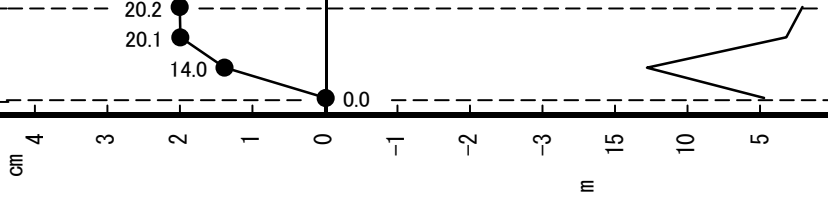
水準点標高断面図
